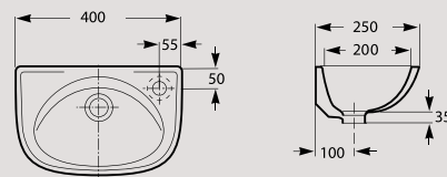
S 1:30 Dimensiuni în mm / E 1:30 Dimensions in mm
